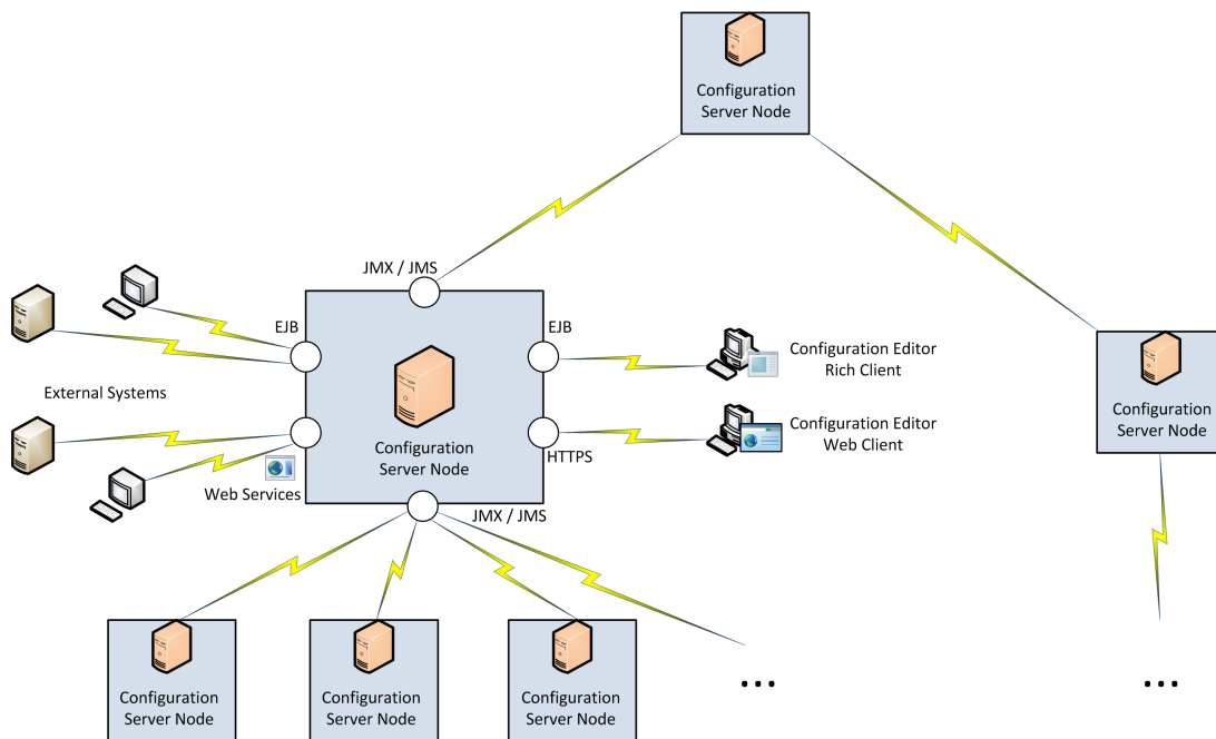
Abbildung 2: Beispielsystem
